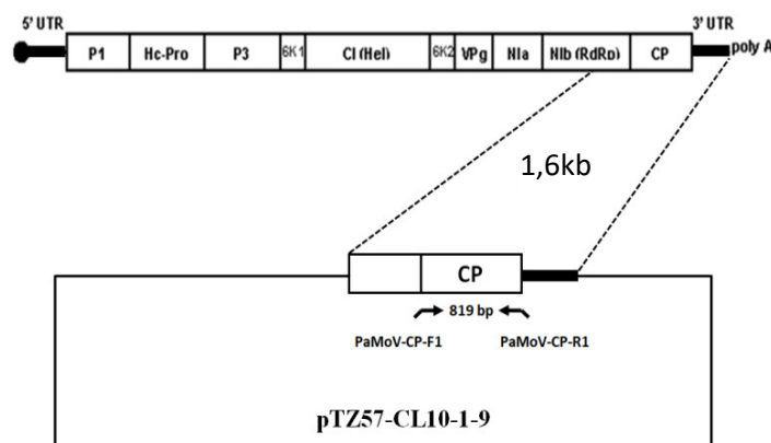
Hình 1. Cấu trúc plasmid pTZ57-CL10-1-9 mang toàn bộ gen mã hóa protein CP của PaMoV và vị trí cặp mỗi để nhân toàn bộ gen này
