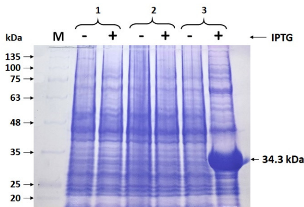
Ghi chú: M là thang protein (GangNam-STAIN™ Prestained Protein Ladder, iNtRON BIO). Dấu (+) và (-) là có và không bổ sung IPTG. Các cặp giếng: 1) Rosetta (DE3), 2) Rosetta (DE3) mang vector pET28a, 3) Rosetta (DE3) mang cấu trúc pET-PaMoV-CP-1. Băng sản phẩm protein tái tổ hợp mong muốn 34,3kDa được chỉ bằng mũi tên.
