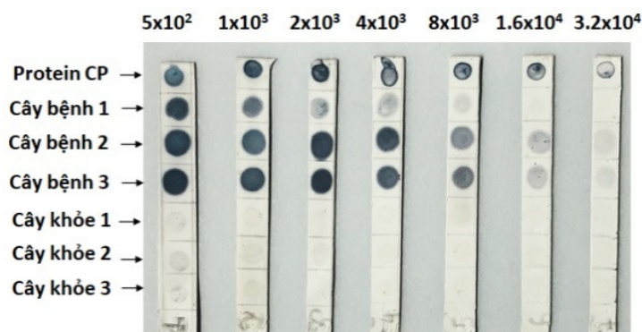
Hình 5. Đánh giá sự hình thành kháng thể đặc hiệu PaMoV trong kháng huyết thanh thô được gây miễn dịch với protein CP tái tổ hợp bằng DIBA
