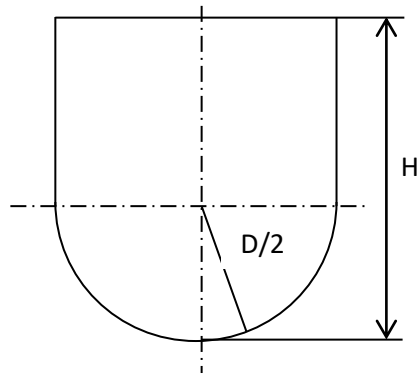
Hình 6. Thùng trộn
